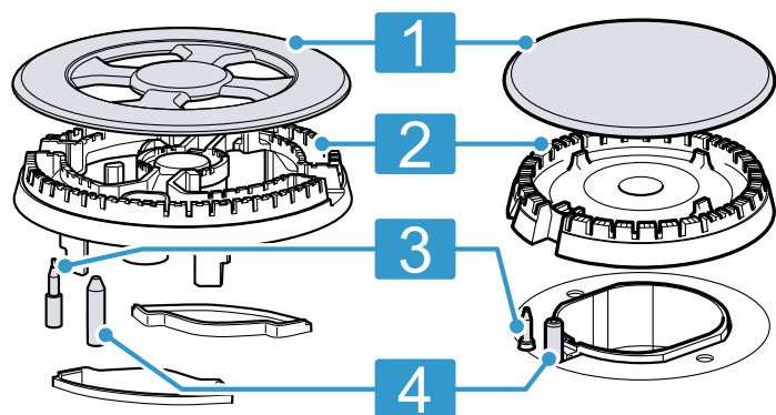
3 Thermoelement für die Flammenüberwachung
